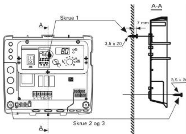
Fig. 26 Vægmontering af kontrolpanelet
