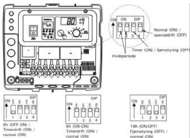
Fig. 28 Indstillingsalternativer for tænd tider.
