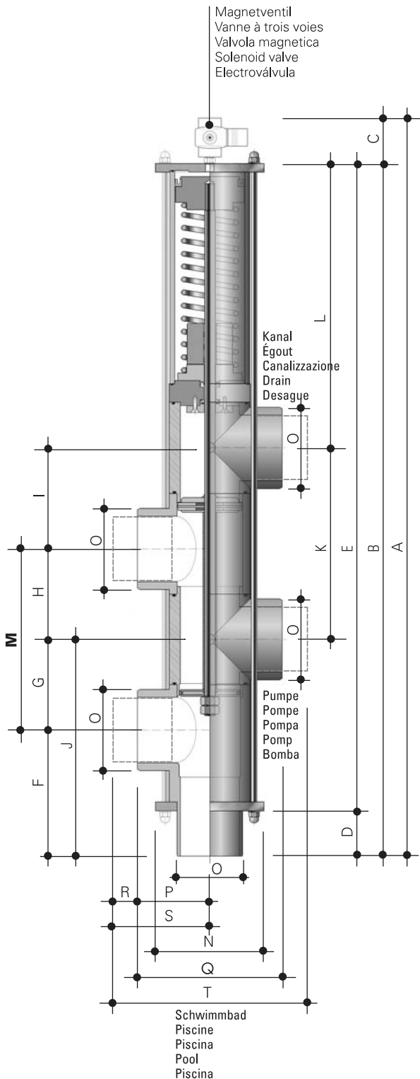
Masstabelle / dimensions / dimensioni / dimensiones
